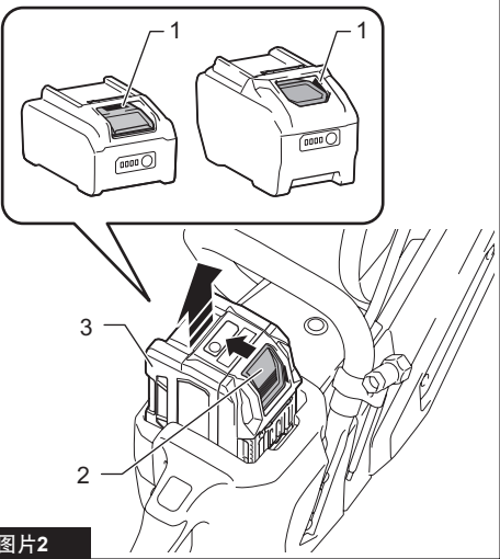
▶ 1. 红色指示器 2. 按钮 3. 电池组
