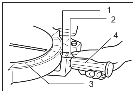
► 1. 指针 2. 锁定杆 3. 等径刻度 4. 手柄
