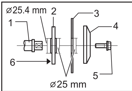
► 1. 主轴 2. 内法兰盘 3. 锯片 4. 外法兰盘 5. 六角螺栓 6. 25.4 mm标记
