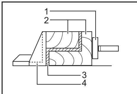
► 1. 水平虎钳 2. 垫块 3. 铝挤压件 4. 导板导向板
