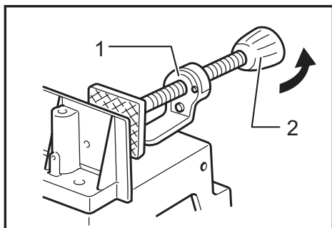
► 1. 凸起部分 2. 虎钳旋钮
