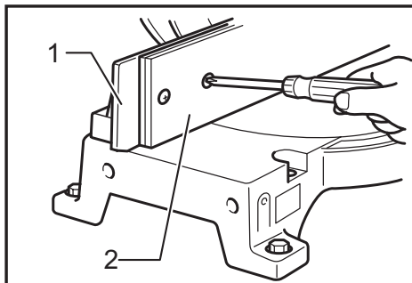
► 1. 导板导向板 2. 木衬片
