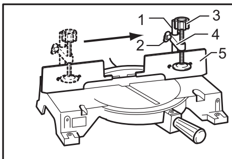
► 1. 虎钳杆 2. 螺丝 3. 虎钳旋钮 4. 虎钳臂 5. 导板导向板
