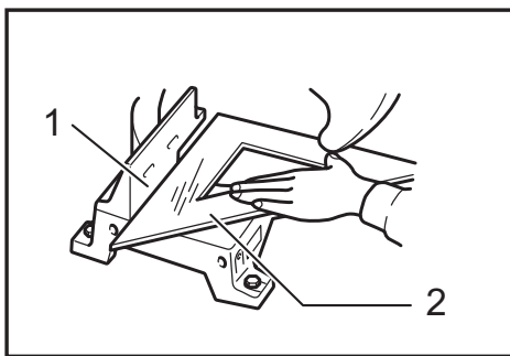
► 1. 导板导向板 2. 三角规
