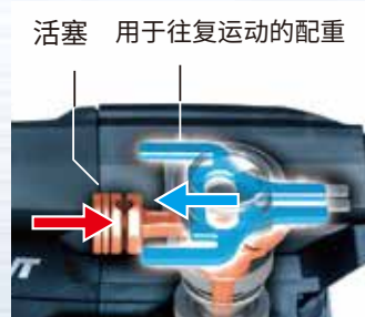
用于往复运动的配重 配重，以消除锤击引起的往复振动
