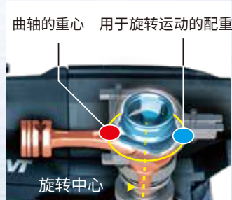
用于旋转运动的配重 配重，用于消除曲轴旋转不平衡引起的振动
