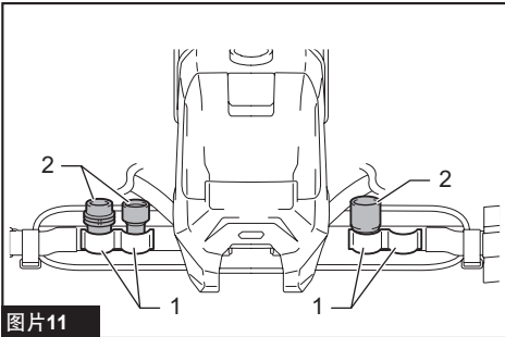
1. 卷环 2. 集尘口
