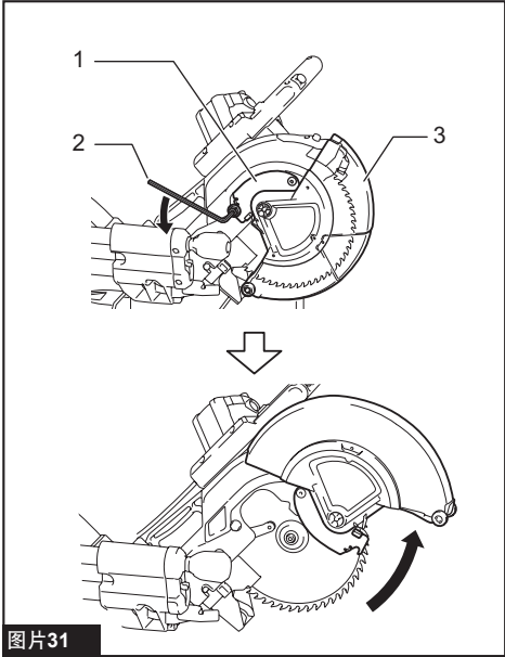
图片31 ► 1. 中心盖板 2. 六角扳手 3. 锯片保护罩
