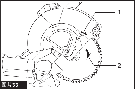
图片33 ► 1. 锯片基座上的箭头 2. 锯片上的箭头
