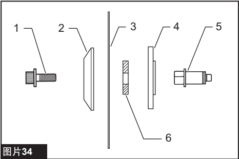
图片34 ► 1. 内六角螺栓 2. 外法兰盘 3. 锯片 4. 内法兰盘 5. 主轴 6. 挡圈
