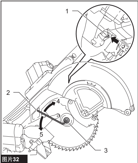
图片32 ► 1. 轴锁 2. 六角扳手 3. 内六角螺栓（左手） 4. 拧松 5. 拧紧
