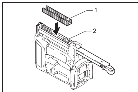
► 1. 马钉 2. 主钉盒
