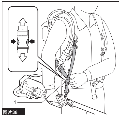
► 1. 带扣
