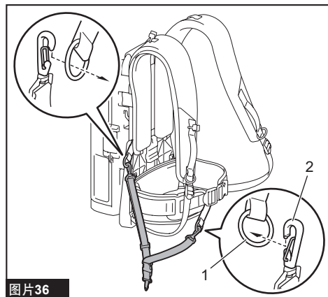
► 1. 挂环 2. 挂钩
