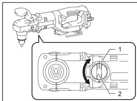
► 1. 指针 2. 变速钮
