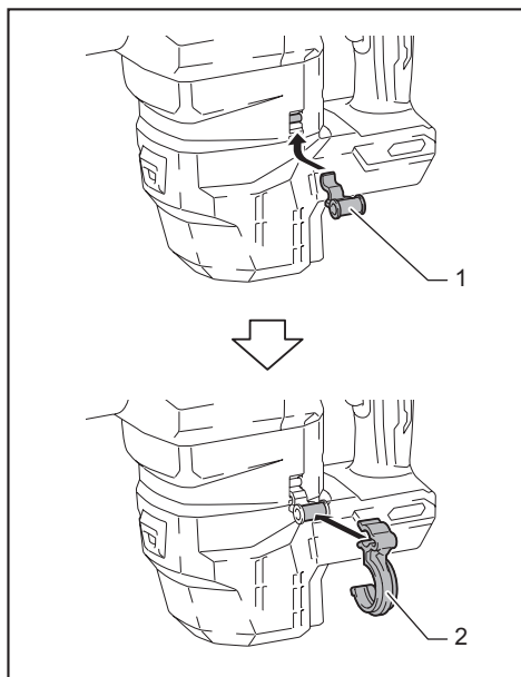
► 1. 托架接头 2. 软管托架 (C)
