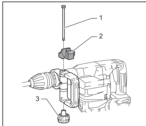
► 1. 六角螺栓 2. 软管托架 (A) 3. 夹紧螺母
