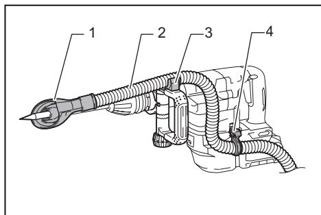
► 1. 防尘罩 2. 软管 3. 软管托架 (A/B) 4. 软管托架 (C)
