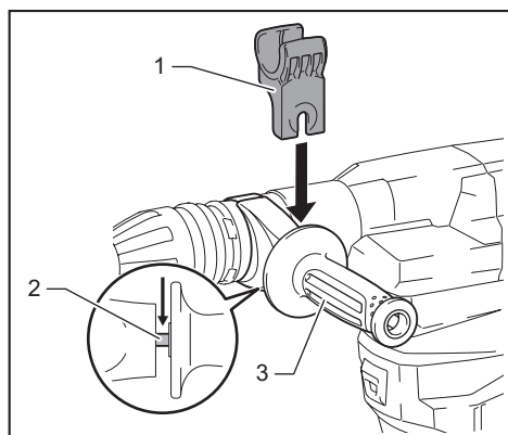
► 1. 软管托架 (B) 2. 轴 3. 侧把手
