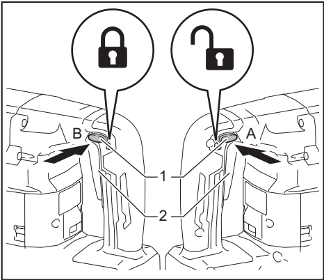
1. 扳机锁按钮 2. 开关扳机
