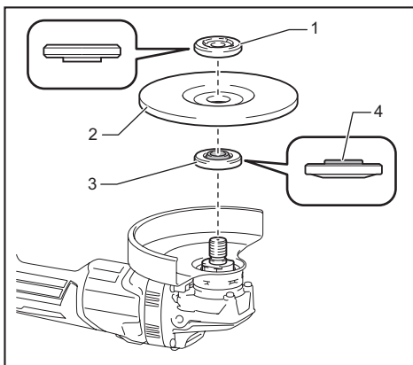
► 1. 锁紧螺母 2. 钹形砂轮 3. 内法兰盘 4. 安装部件
