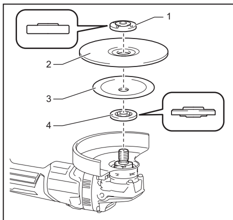
► 1. 锁紧螺母 2. 弹性砂轮片 3. 支撑垫 4. 内法兰盘
