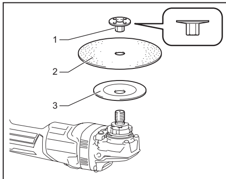
► 1. 砂磨用锁紧螺母 2. 砂轮片 3. 橡胶垫
