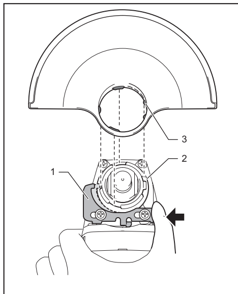
► 1. 锁定杆 2. 槽口 3. 凸起部分
