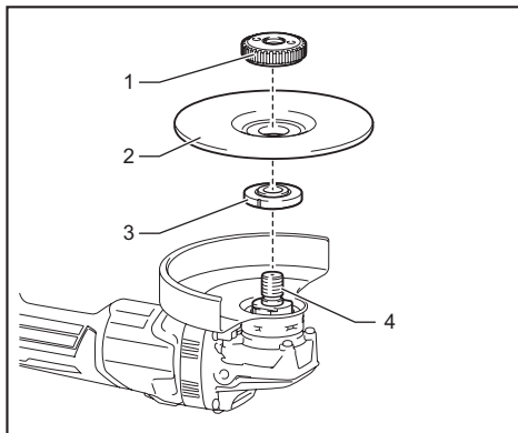
► 1. 使用螺母（Ezynut） 2. 砂轮 3. 内法兰盘 4. 主轴
