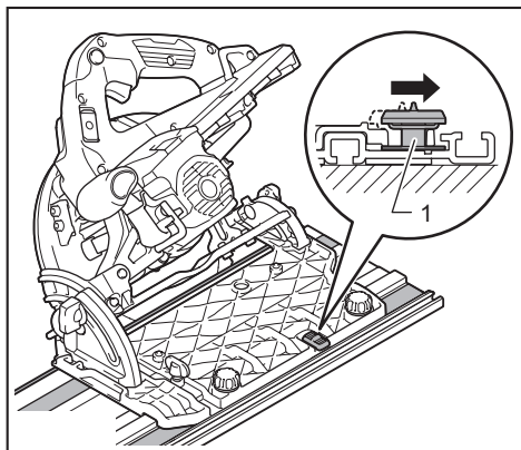
► 1. 滑动杆
