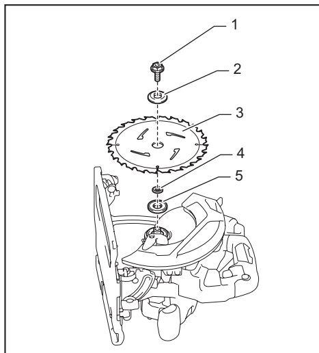
► 1. 六角螺栓 2. 外法兰盘 3. 电动圆锯锯片 4. 挡圈 5. 内法兰盘
