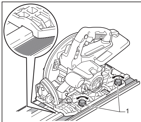
► 1. 调节螺丝
