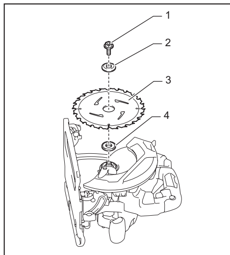
► 1. 六角螺栓 2. 外法兰盘 3. 电动圆锯锯片 4. 内法兰盘
