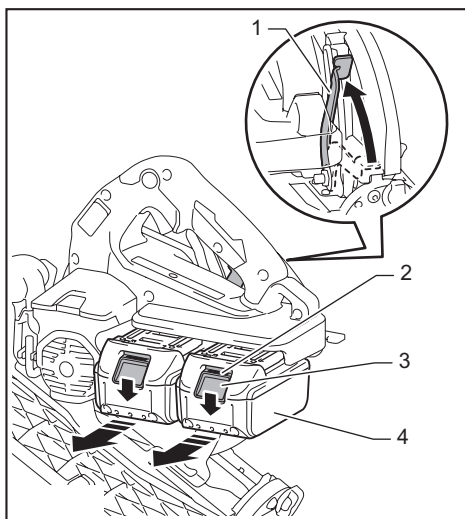
► 1. 杆 2. 红色指示器 3. 按钮 4. 电池组
