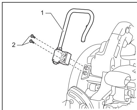
► 1. 挂钩 2. 螺丝
