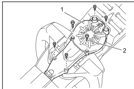
► 1. 护罩 2. 螺栓
