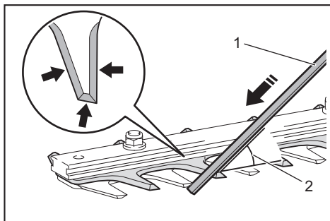
► (1) 锉刀 (2) 45°
