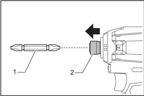
► 1. 起子头 2. 套筒
