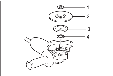
► 1. 锁紧螺母 2. 伸缩轮 3. 支撑垫 4. 内法兰盘
