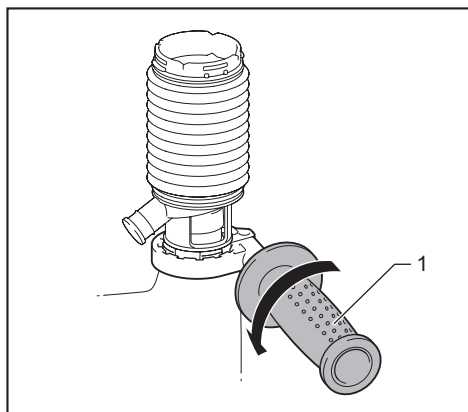
► 1. 侧把手
