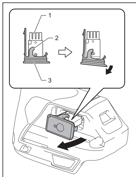
► 1. 无线装置 2. 挂钩 3. 封盖
