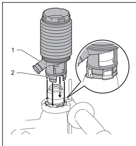
► 1. 集尘杯 2. 卡爪
