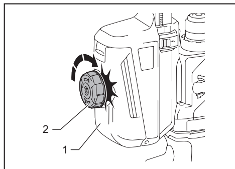
► 1. 集尘盒 2. 拨盘
