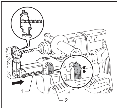
► 1. 导板 2. 导板调节按钮
