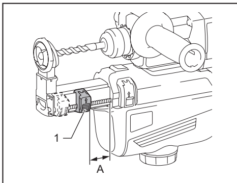
► 1. 深度调节按钮
