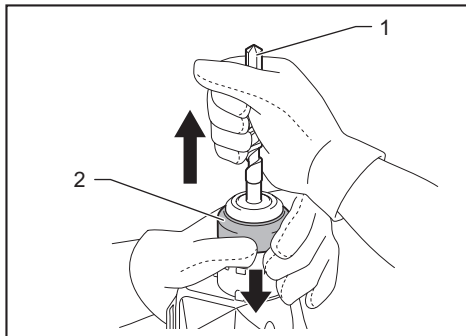
► 1. 钻头 2. 卡盘盖
