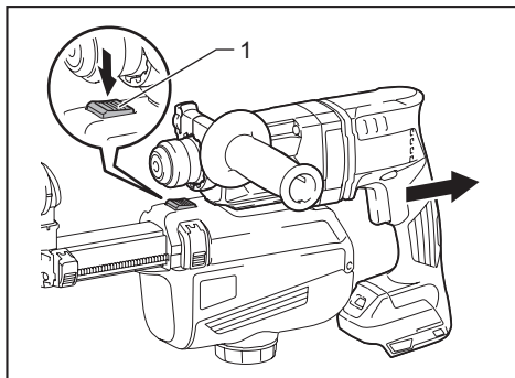
► 1. 锁止按钮
