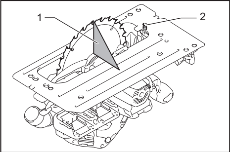
► 1. 三角规 2. 0° 角调节螺丝
