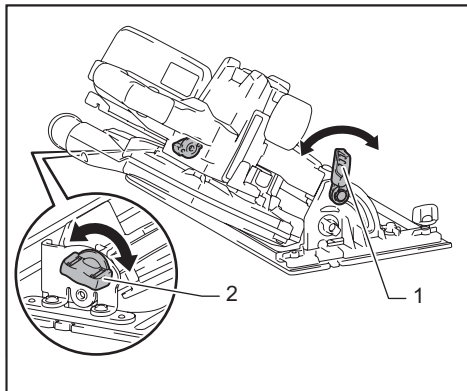
► 1. 杆 2. 夹紧螺丝
