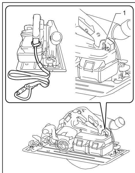
► 1. 系索（系带）用孔
