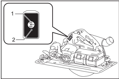
► 1. 无线启动按钮 2. 无线启动指示灯
