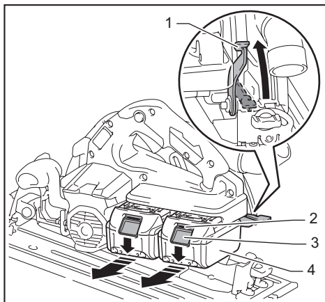
► 1. 杆 2. 红色指示器 3. 按钮 4. 电池组
