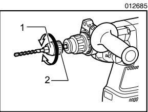
1. 套筒 2. 挡圈
