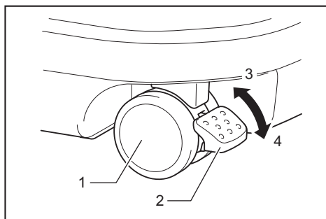
► 1. 脚轮 2. 止动杆 3. 自由位置 4. 锁定位置
