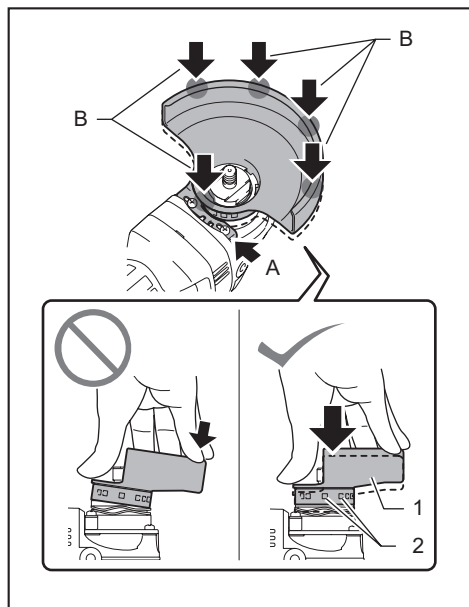
► 1. 砂轮罩 2. 孔
