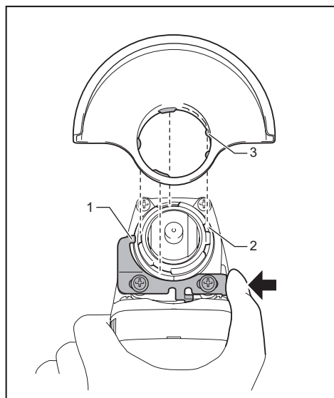
► 1. 锁定杆 2. 槽口 3. 凸起部分
