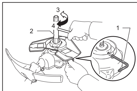
► 1. 六角扳手 2. 套筒扳手 3. 拧紧 4. 拧松
