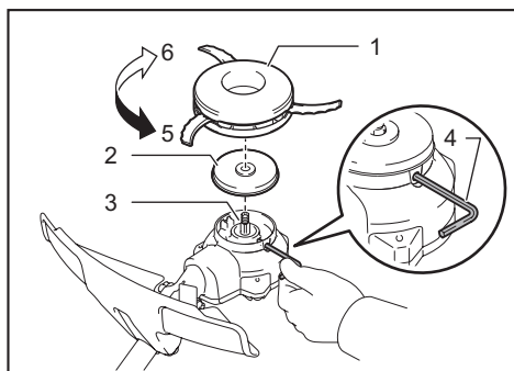
► 1. 塑料刀片 2. 挡圈 3. 主轴 4. 六角扳手 5. 拧紧 6. 拧松
