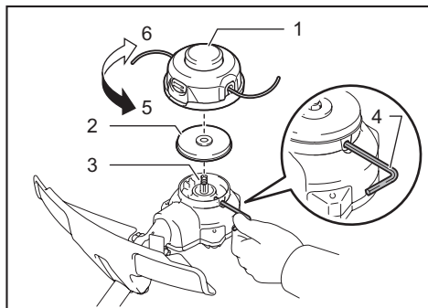
► 1. 尼龙打草头 2. 挡圈 3. 主轴 4. 六角扳手 5. 拧紧 6. 拧松
