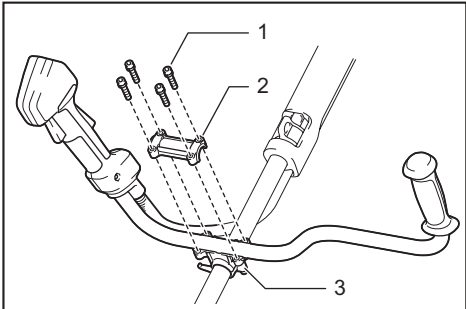
► 1. 内六角头螺栓 2. 把手夹 3. 把手托架
