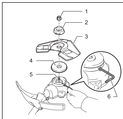
► 1. 螺母 2. 锁紧垫圈 3. 刀片 4. 挡圈 5. 主轴 6. 六角扳手
