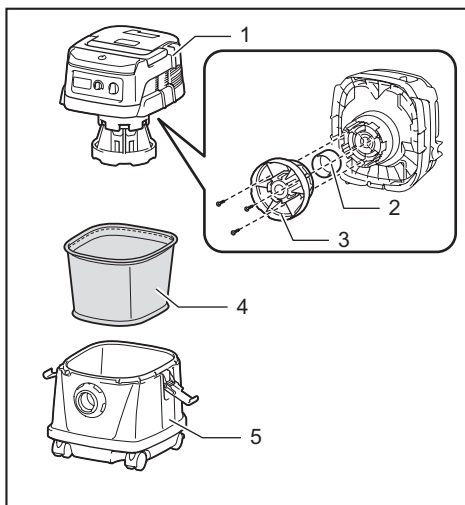
► 1. 容器盖 2. 浮标 3. 浮标套筒 4. 布质过滤器 5. 容器
