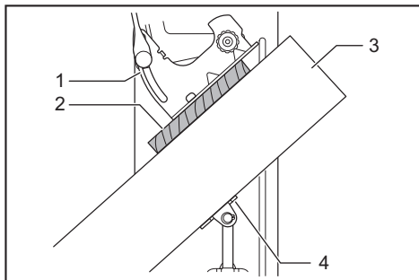
► 1. 导向板 2. 垫块（超过190 mm长 x 40 mm宽） 3. 工件（超过85 mm宽） 4. 虎钳板
