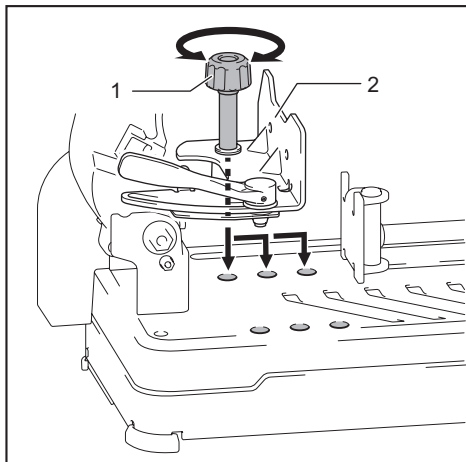
► 1. 螺丝 2. 导向板
