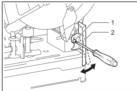
► 1. 螺丝 2. 火花罩
