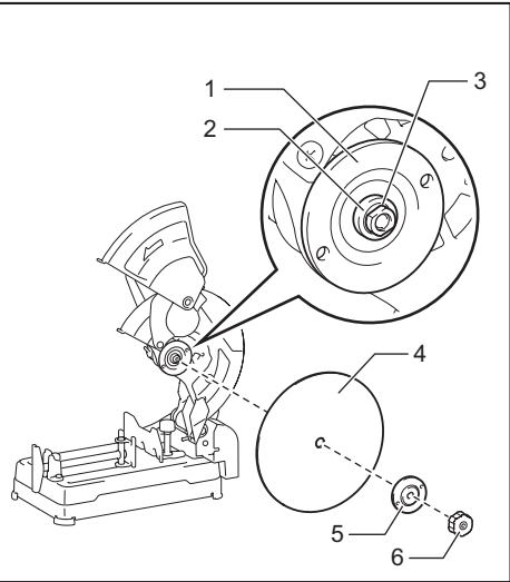
► 1. 内法兰盘 2. 挡圈 3. O形环 4. 切割砂轮 5. 外法兰盘 6. 免工具夹
