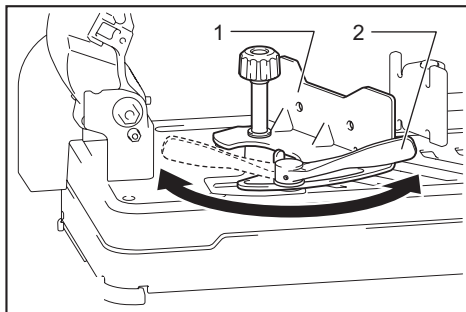
► 1. 导向板 2. 杆
