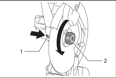
► 1. 轴锁 2. 免工具夹
