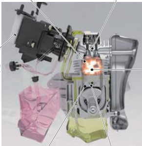
连杆两端使用滚针轴承
