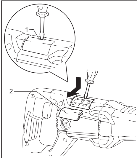
▶ 1. 槽口 2. 护盖
