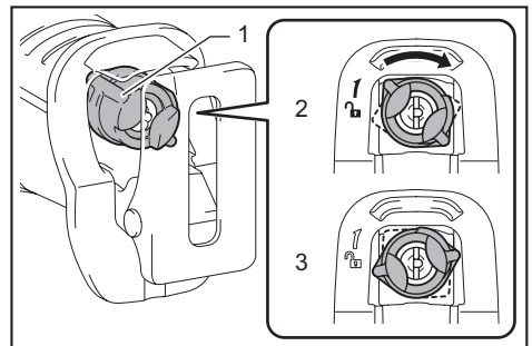
▶ 1. 锯片夹杆 2. 释放位置 3. 固定位置
