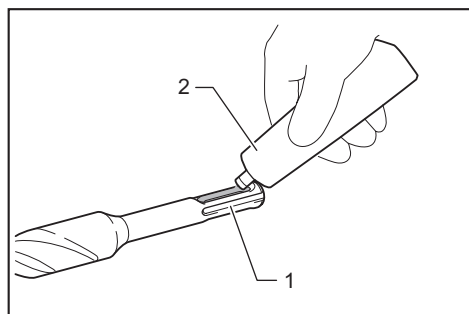
► 1. 柄端 2. 润滑脂
