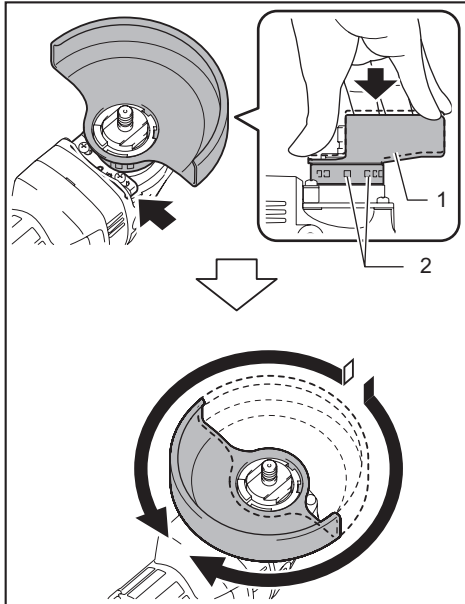
▶ 1. 砂轮罩 2. 孔
