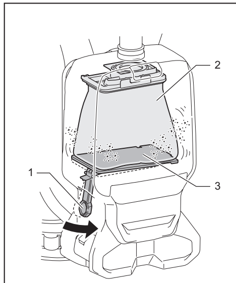
► 1. 拉杆 2. 过滤袋/集尘袋 3. 平板
