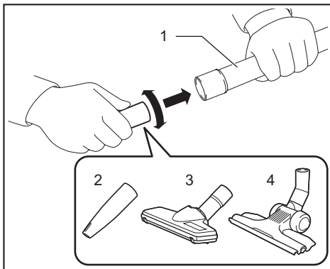
► 1. 伸延杆 2. 通用集尘口 3. T型集尘口 4. T型集尘口（纤细）
