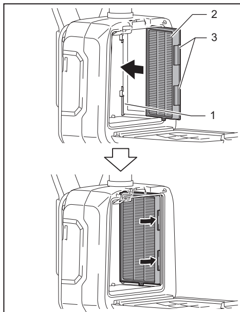
► 1. 凹槽 2. HEPA过滤器 3. 挂钩
