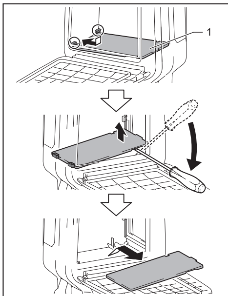
► 1. 平板
