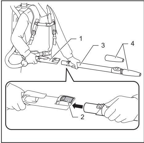
► 1. 弯管组件 2. 按钮 3. 滑动型伸延杆 4. 通用集尘口
