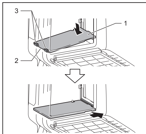
► 1. 平板 2. 直边 3. 搭扣
