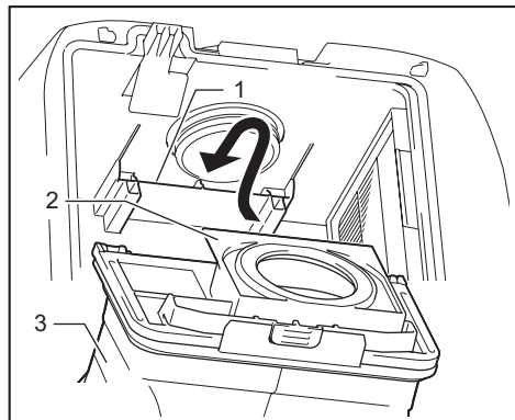
► 1. 凹槽 2. 边缘 3. 集尘袋
