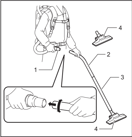
► 1. 38号前端管口 2. 铝弯管 3. 铝直管 4. 集尘口
