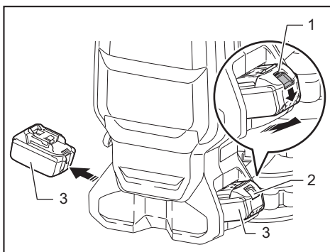
► 1. 红色指示灯 2. 按钮 3. 电池组
