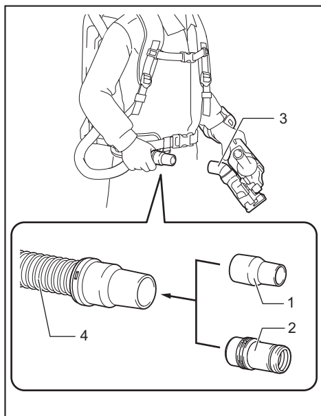
► 1. 接头 2. 前端管口 3. 除尘出气口 4. 软管
