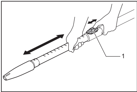
► 1. 滑动钮
