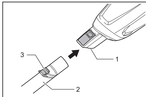
► 1. 吸气口 2. 伸缩杆 3. 卡钩
