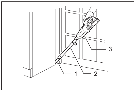
► 1. 角落集尘口 2. 伸延杆 3. 吸尘机主机
