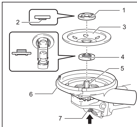
► 1. 锁紧螺母 2. 凸出部分 3. 偏置金刚石砂轮 4. 内法兰盘 5. 主轴 6. 偏置式金刚石砂轮适用的集尘式砂轮罩 7. 轴锁
