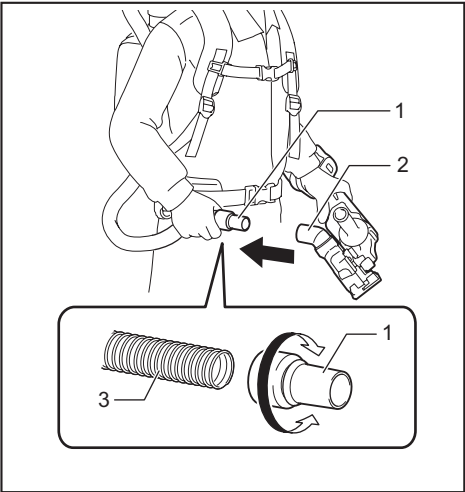
► 1. 前端管口 2. 除尘出口口 3. 软管
