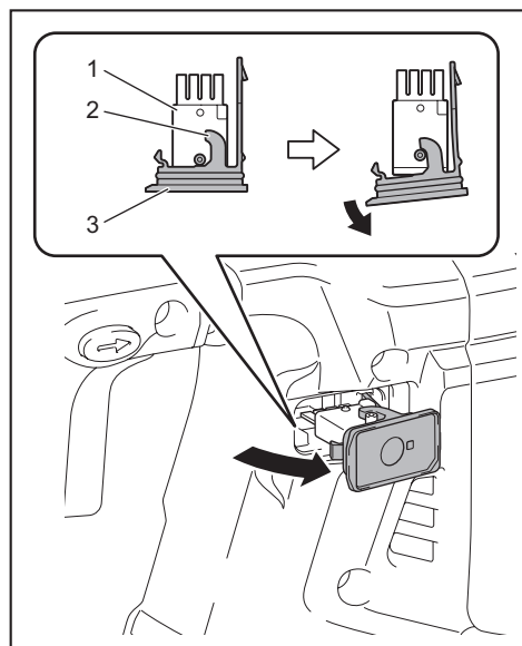
► 1. 无线装置 2. 挂钩 3. 封盖
