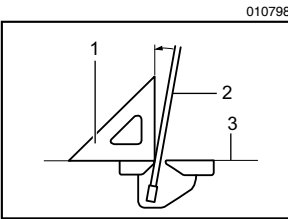
1. 三角规 2. 锯片 3. 翻转台的顶面
