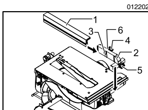
1. 切锯导板 2. 切锯导板座 3. 方形螺母 4. 夹紧螺丝（A） 5. 夹紧螺丝（B） 6. 垫圈
