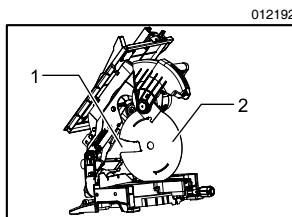
1. 锯片保护罩 B 2. 锯片
