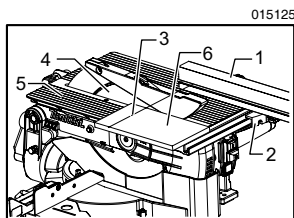
1. 切锯导板 2. 切锯导板座 3. 要对齐的线 4. 锯片 5. 上部工作台 6. 工件
