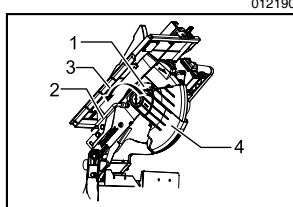
1. 中心盖板 2. 套筒扳手 3. 六角螺栓 4. 下部锯片保护罩 A
