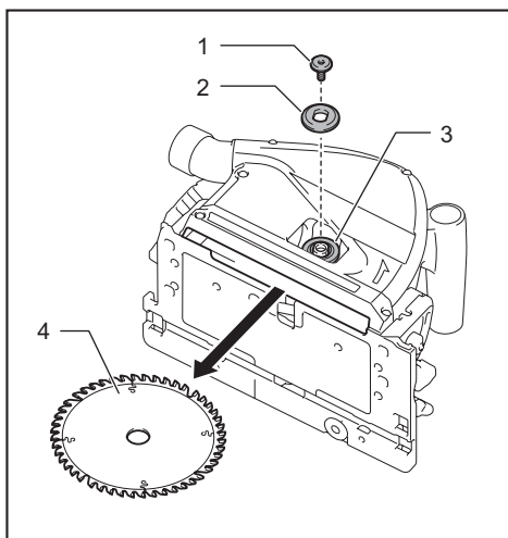
► 1. 六角螺栓 2. 外法兰盘 3. 内法兰盘 4. 电圆锯锯片
