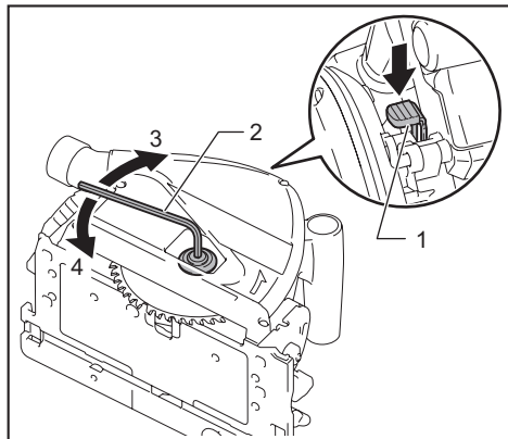
► 1. 轴锁 2. 六角扳手 3. 拧紧 4. 拧松
