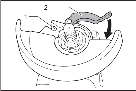
► 1. 螺丝 2. 杆
