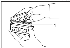
1. 刨刀夹
