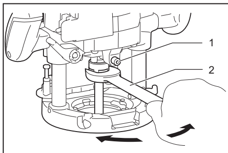
► 1. 轴锁 2. 扳手
