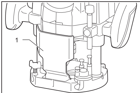
► 1. 碎屑挡板
