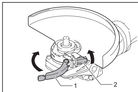
► 1. 杆 2. 螺母
