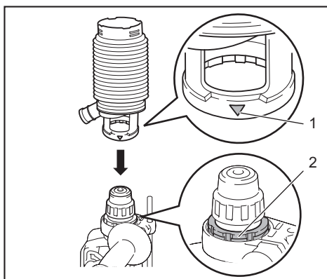
► 1. △符号 2. 凹槽
