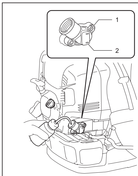
► 1. 上限标记 2. 下限标记
