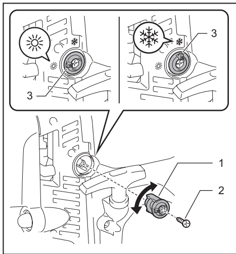
► 1. 除雾杆 2. 螺丝 3. 点
