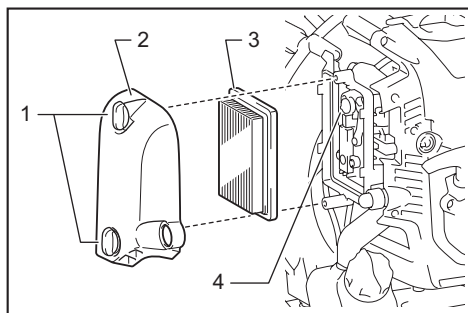
► 1. 旋钮螺栓 2. 空气过滤器盖 3. 组件 4. 通气阀
