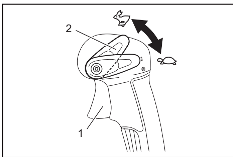
► 1. 油门扳机 2. 停止控制杆
