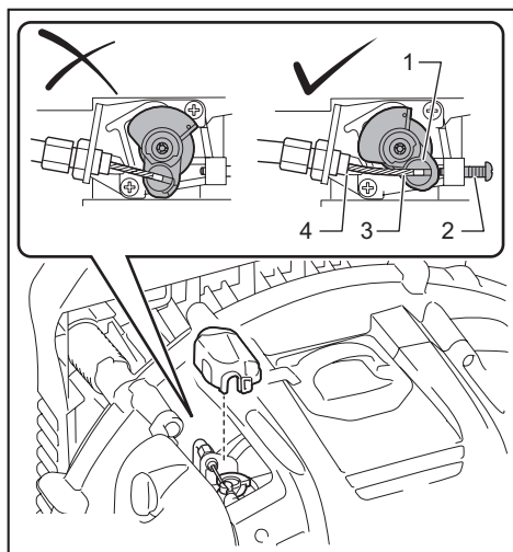
► 1. 油门阀 2. 怠速调节螺丝 3. 控制线索 4. 油门阀止动器
