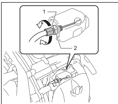
► 1. 线索调节螺栓 2. 固定螺母
