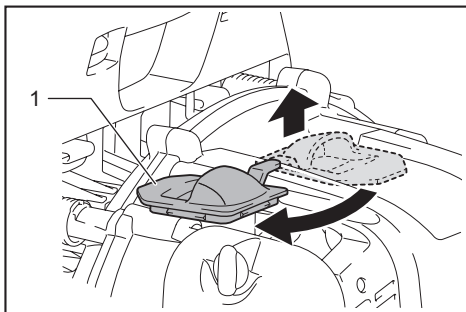
► 1. 火花塞盖
