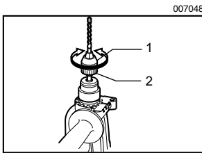
1. 套筒 2. 挡圈
