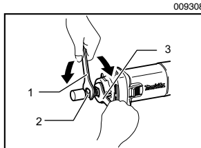
1. 13号扳手 2. 筒夹螺母 3. 13号扳手
