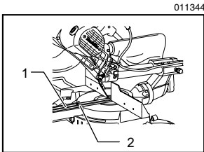
1. 锯槽板 2. 螺丝
