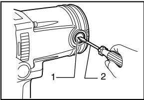
1. 碳刷夹盖子
