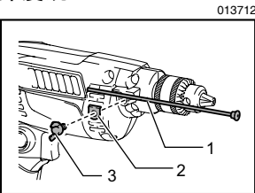
1. 深度规 2. 垫圈 3. 夹紧螺丝
