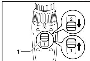
1. 变速拨杆
