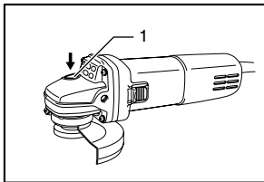
1. 转轴锁定器
