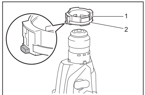
► 1. 衬套 2. 弹簧
