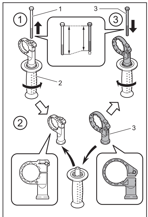
► 1. 螺栓 2. 把手 3. 选购件把手基座组件
