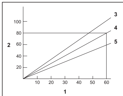
1. 射钉频率 (次/min) 2. 压缩机每分钟空气输出量 (L/min) 3. 0.83 MPa (8.3 bar) 4. 0.66 MPa (6.6 bar) 5. 0.49 MPa (4.9 bar)
