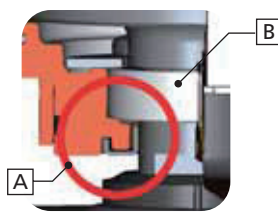
A 迷宫式密封防护结构 B 防尘滚珠轴承
