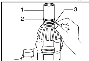
1. 套筒 2. O 形圈 3. 销
