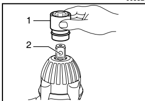
1. 套筒 2. 砧座
